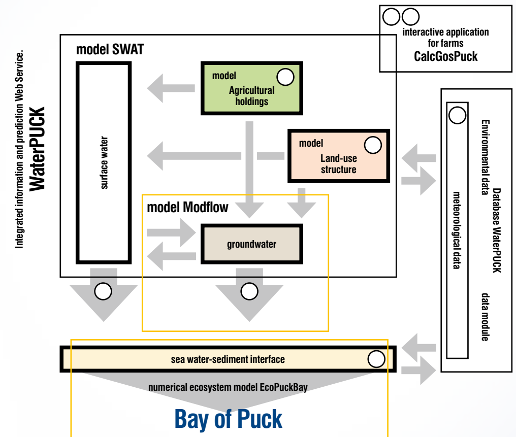
Schemat Zintegrowanego Serwisu informacyjno-predykcijnego WaterPUCK, Przepływ informacji poprzez poszczególne moduły Serwisu
