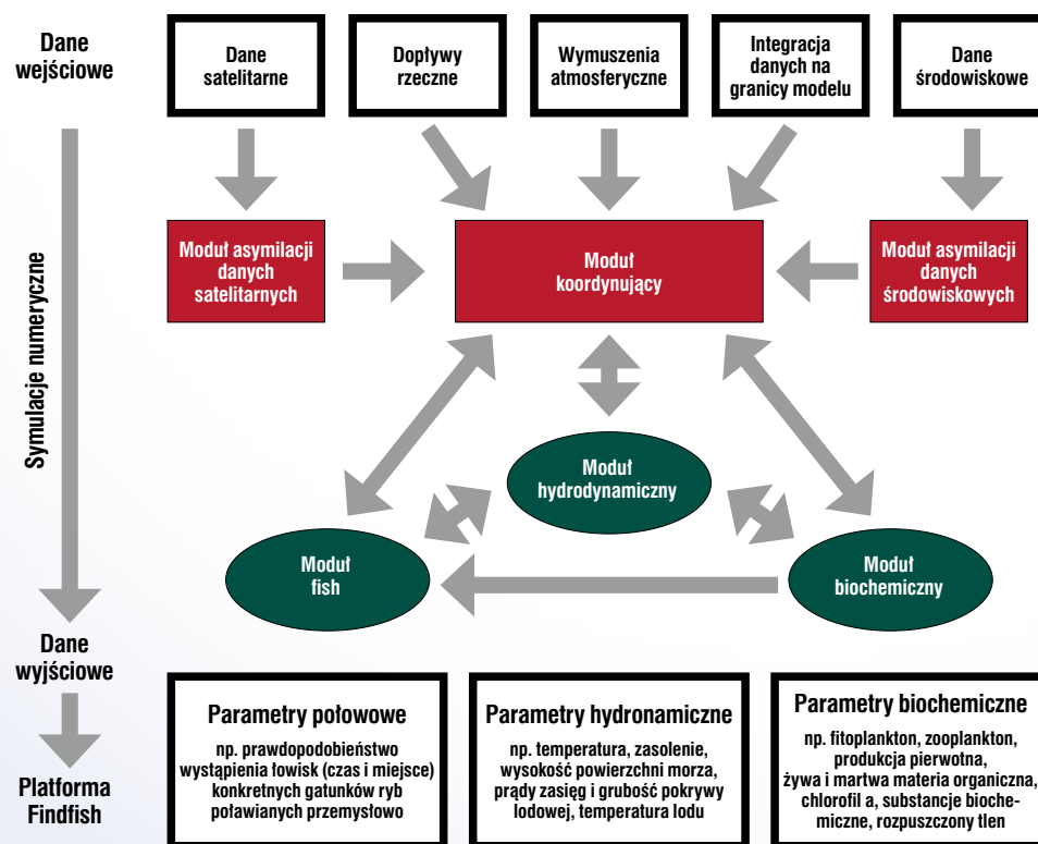
Schemat Modelu ekohydrodynamicznego EcoFish z modulem Fish
